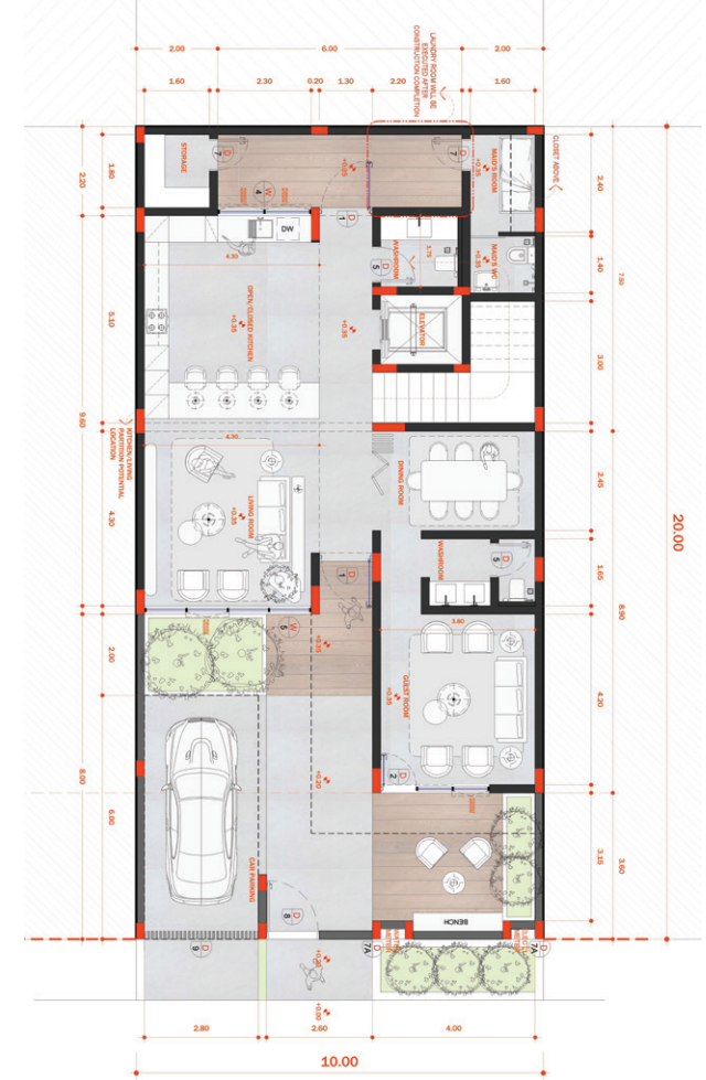
الدور الأرضي
