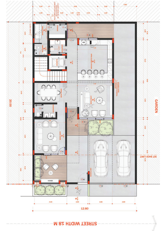
الدور الأرضي
