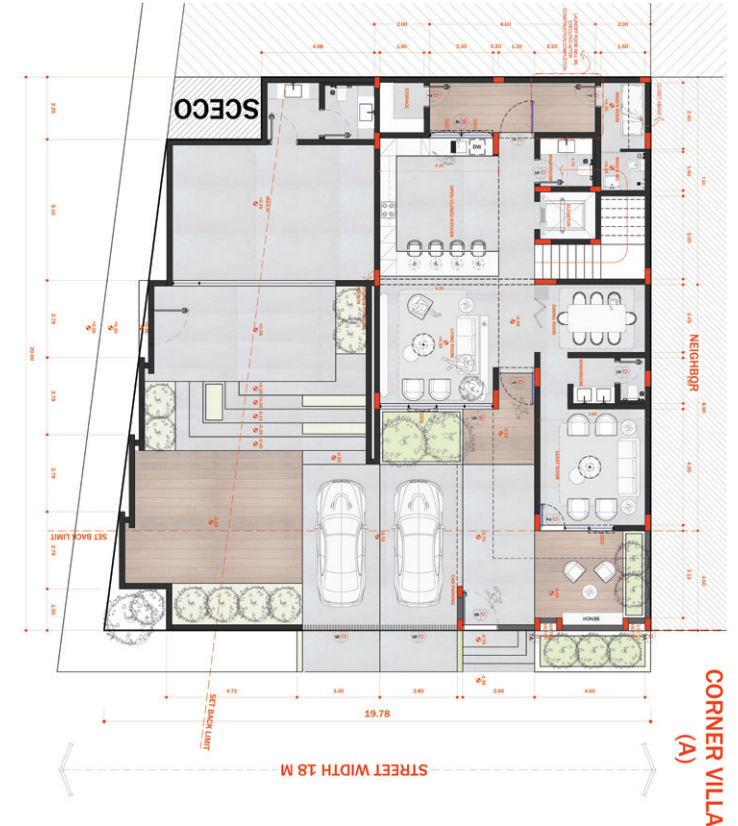
الدور الأرضي
