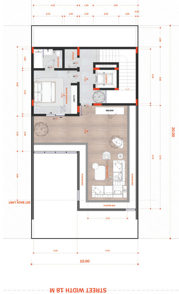
الدور الملحق
