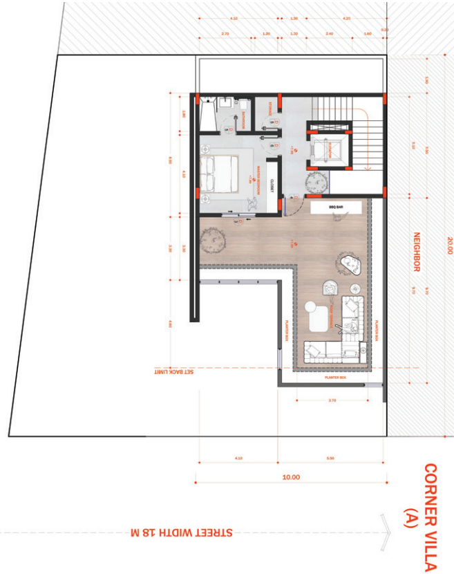
الدور الملحق
