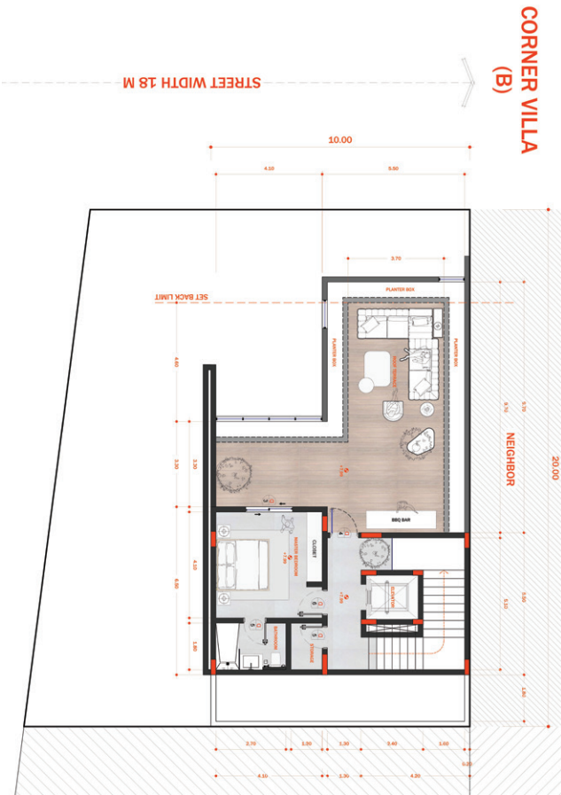
الدور الملحق
